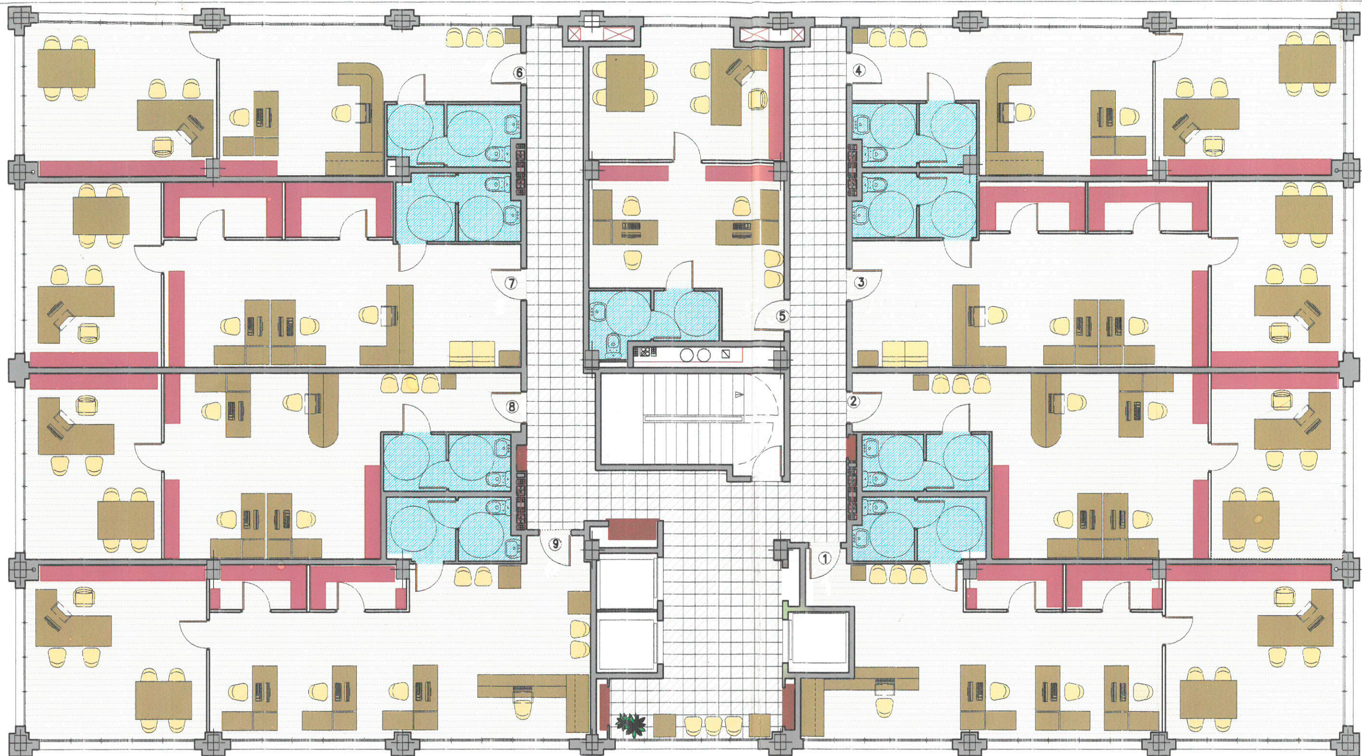
PLANTA PRIMERA
